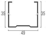
DC 50 profili (35 x 35)
